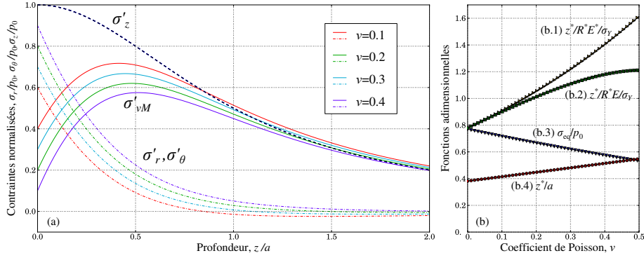
Figure 1.7. (a) Contraintes \sigma_\theta , \sigma_r et \sigma_z le long de l'axe de symétrie ; (b) des fonctions adimensionnelles qui représentent (b.1) la profondeur normalisée de commencement d'écoulement plastique z^*/R^*E^*/\sigma_Y , (b.2) la profondeur normalisée dans le cas d'indenteur rigide z^*/R^*E^*/\sigma_Y , (b.3) la contrainte de von Mises maximale normalisée \sigma_{eq}/p_0 , (b.4) la profondeur normalisée z^*/a , la solution d'Eq. [1.16] ; les lignes solides dans (b) représentent des solutions approximatives [1.19],[1.20],[1.18],[1.17], respectivement.
