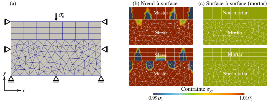
Figure 1.5. Comparaison des contraintes normales \sigma_{yy} dans le cas de discrétisation (b) nœud-à-surface (NTS) et (c) surface-à-surface (STS) pour des différents choix des surfaces maître-esclave (master-slave) et mortier – non-mortier dans les cas NTS et STS, respectivement (figure adaptée de (Akula 2019)).
